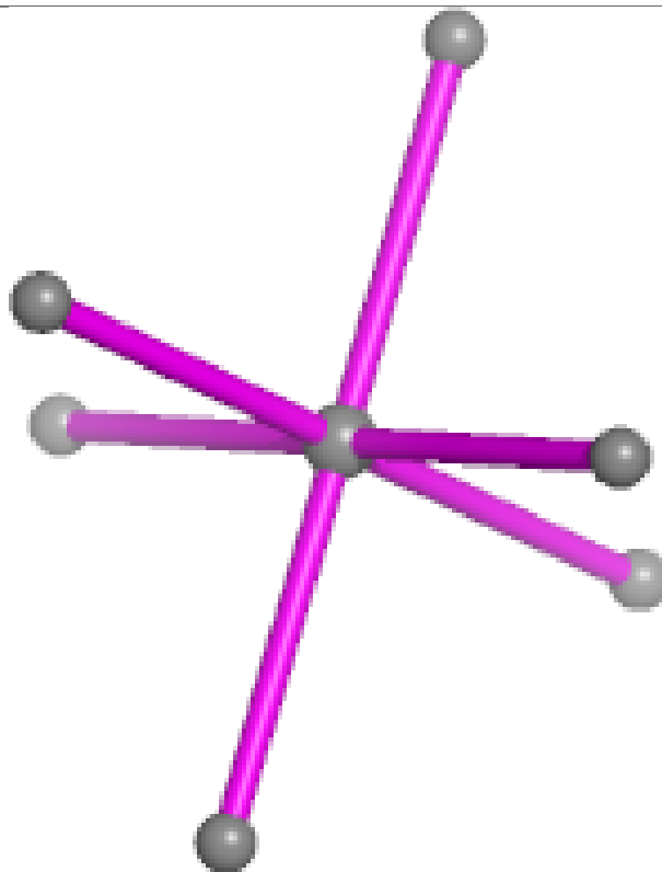
Bond angles
