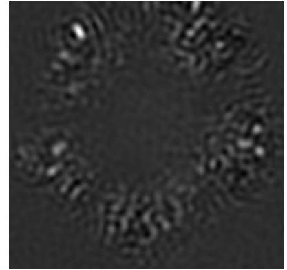
Z Index: 201
